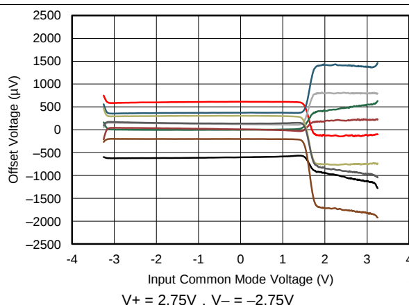
图 4. 失调电压与共模电压间的关系
