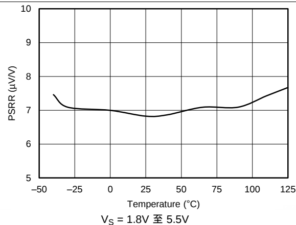
图 14. PSRR 与温度间的关系
