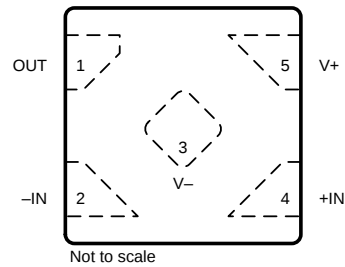
引脚功能：TLV9061
