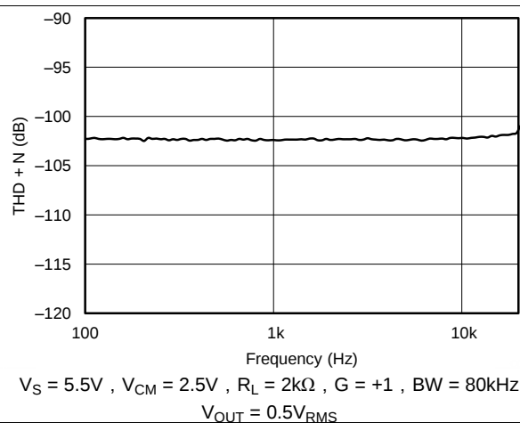
图 17. THD + N 与频率间的关系
