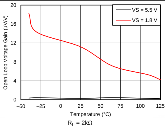
图 7. 开环增益与温度间的关系
