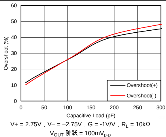
图 24. 小信号过冲与负载电容间的关系
