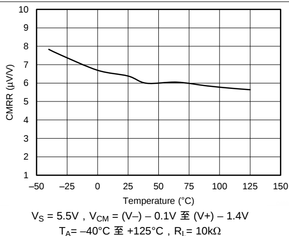
图 13. CMRR 与温度间的关系
