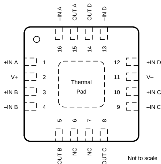
引脚功能：TLV9064
