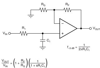
单极低通滤波器
