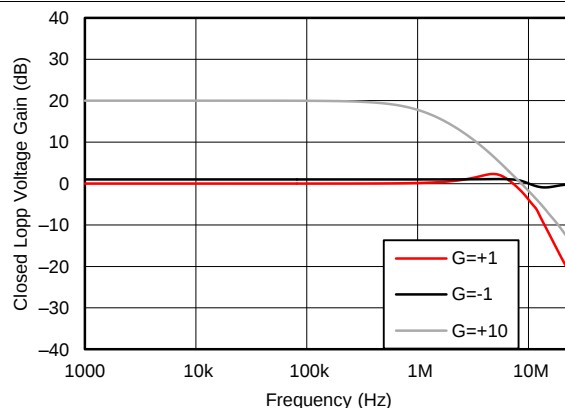
图 8. 闭环增益与频率间的关系
